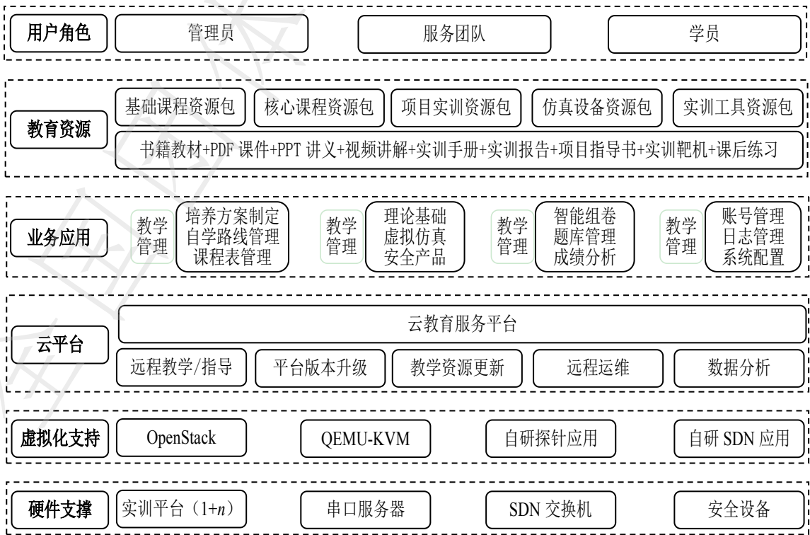
图7 实训室平台系统结构图
